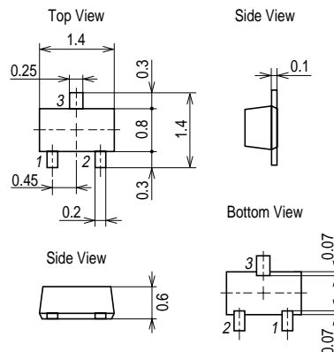
外形図 2159A (unit: mm)
