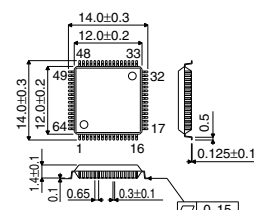
SQFP-T64
