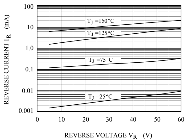
I_R - V_R
