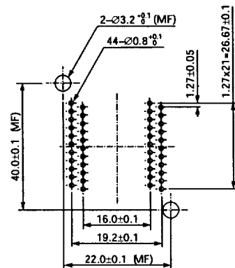
SOP IC51-0442-1315 (44 Pins)
