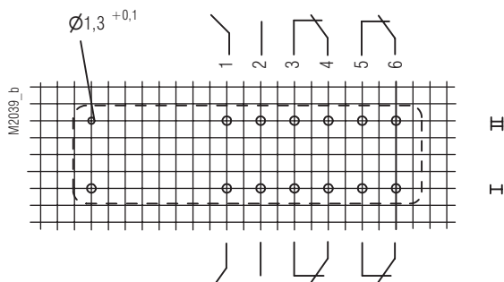
Connexions des picots OA 5612.50/...L1 2NO / 4NF
