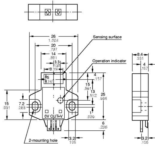
UZJ111 UZJ112 Sensor
