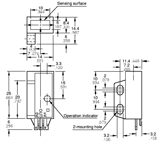
UZJ261 UZJ262 Sensor
