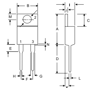
TO-220A
