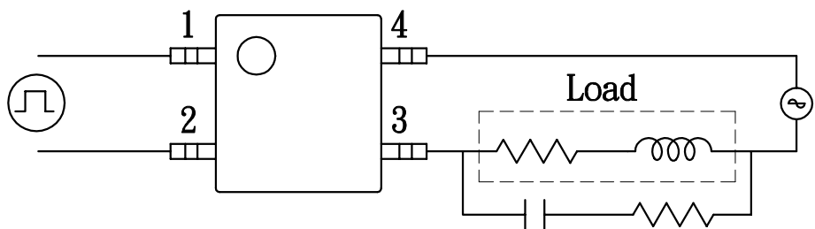
R-C Snubber
