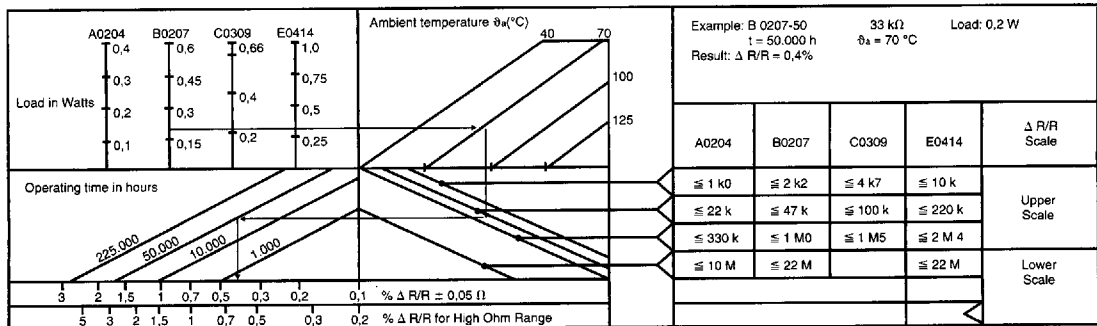
Fig. 5 Nomogram
