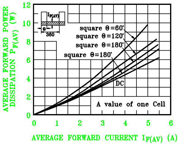
P_{F(AV)} - I_{F(AV)}
