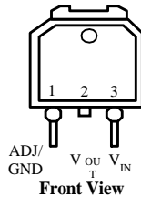
TO-252 (D)
