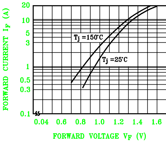
I_F - V_F
