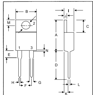
TO-220A
