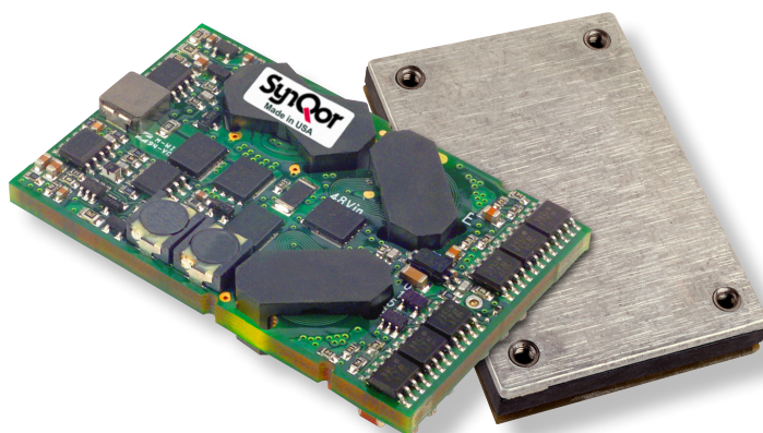
PQ40150QGx07 Module
