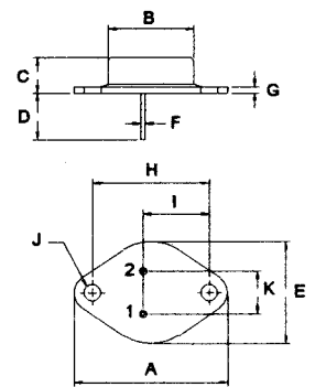
TO-3
