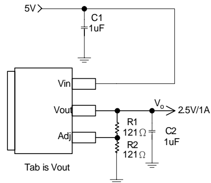
( 5V/2.5V ADJ output )
